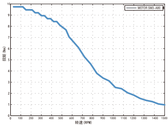
电机型号: SM3-A80 测试条件: 细分设置1000P/R 驱动器型号: SD3228 驱动器电流: 6.4A 供电电压: 220VAC
