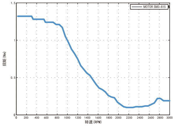
电机型号: SM3-615 驱动器型号: SD388 供电电压: 36VDC 测试条件: 细分设置1000P/R 驱动器电流: 8A
