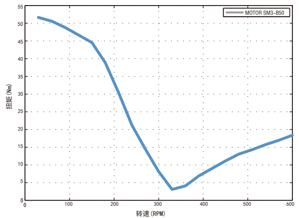
电机型号: SM3-B50 测试条件: 细分设置1000P/R 驱动器型号: SD3228 驱动器电流: 5.6A 供电电压: 220VAC
