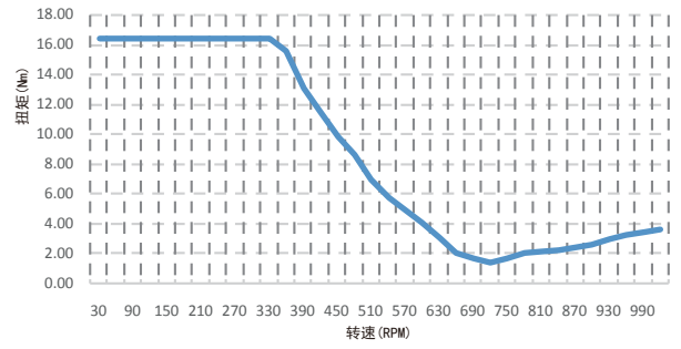
电机型号: SM3-B20A 测试条件: 细分设置1000P/R 驱动器型号: SD3228N 驱动器电流: 5.6A 供电电压: AC220V
