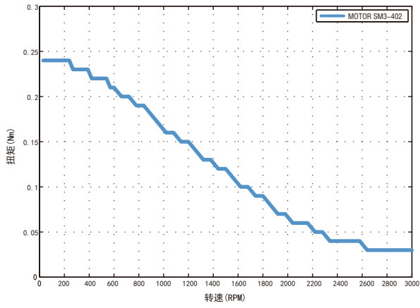
电机型号: SM3-402 驱动器型号: SD366 供电电压: 36VDC 测试条件: 细分设置1000P/R 驱动器电流: 2.1A
