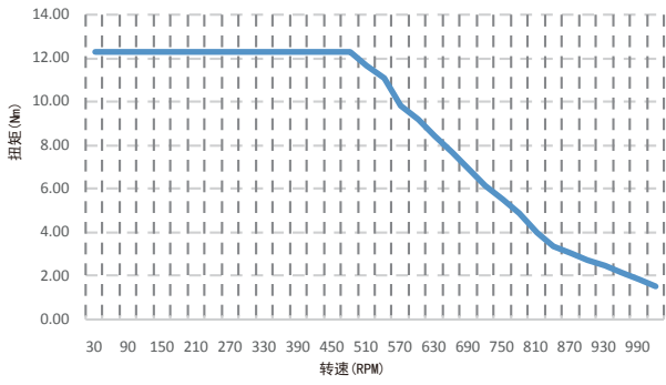
电机型号: SM3-B15A 测试条件: 细分设置1000P/R 驱动器型号: SD3228N 驱动器电流: 5.6A 供电电压: AC220V
