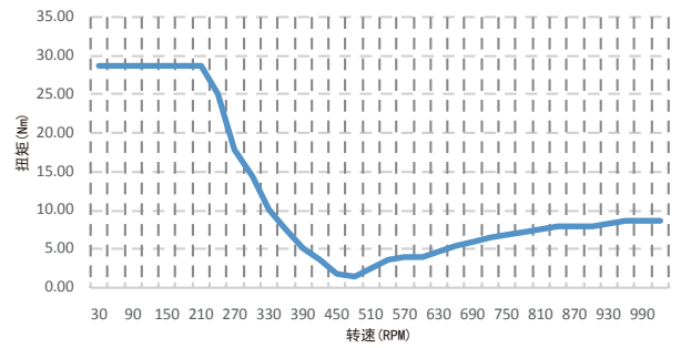
电机型号: SM3-B35A 测试条件: 细分设置1000P/R 驱动器型号: SD3228N 驱动器电流: 5.6A 供电电压: AC220V
