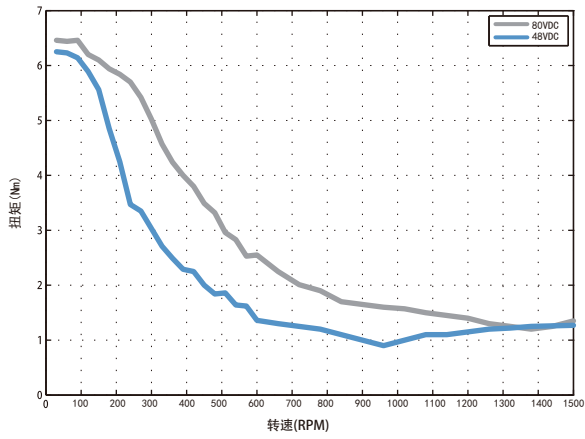
电机型号: SM3-960 测试条件: 细分设置1000P/R 驱动器型号: SD388 驱动器电流: 8A 供电电压: 见图
