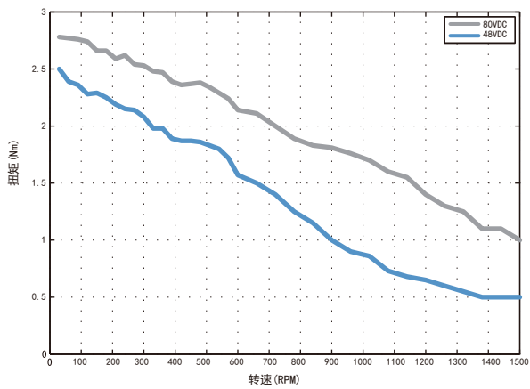
电机型号: SM3-920 驱动器型号: SD388 供电电压: 见图 测试条件: 细分设置1000P/R 驱动器电流: 8A
