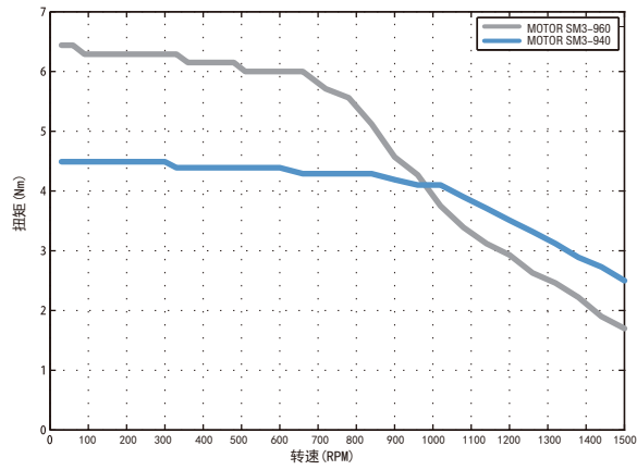
电机型号: SM3-940/960 测试条件: 细分设置1000P/R 驱动器型号: SD3228 驱动器电流: 8A 供电电压: 220VAC
