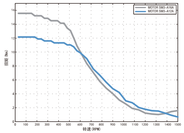
电机型号: SM3-A12A/A16A 测试条件: 细分设置1000P/R 驱动器型号: SD3228 驱动器电流: 8A 供电电压: 220VAC
