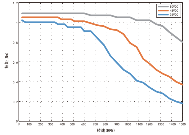
电机型号: SM3-609 驱动器型号: SD388 供电电压: 见图 测试条件: 细分设置1000P/R 驱动器电流: 8A
