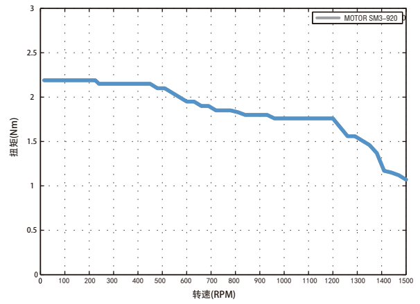
电机型号: SM3-920 测试条件: 细分设置1000P/R 驱动器型号: SD3228 驱动器电流: 8A 供电电压: 220VAC
