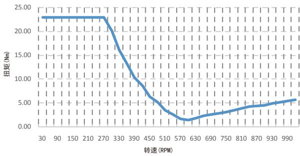
电机型号: SM3-B28A 测试条件: 细分设置1000P/R 驱动器型号: SD3228N 驱动器电流: 5.6A 供电电压: AC220V
