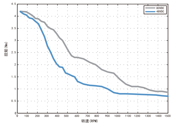
电机型号: SM3-940 驱动器型号: SD388 供电电压: 见图 测试条件: 细分设置1000P/R 驱动器电流: 8A
