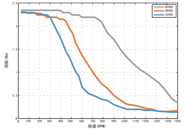
电机型号: SM3-620 驱动器型号: SD388 供电电压: 见图 测试条件: 细分设置1000P/R 驱动器电流: 8A
